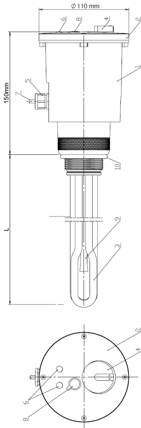
Abb.1 Aufbau der Heizpatrone.
