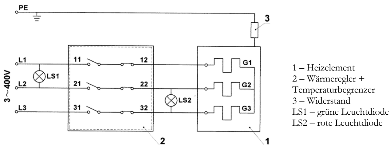
Abb. 2 Das elektrische Schema
